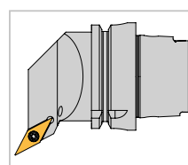
HSK-T63- SV117,5CL/R 45070-16
