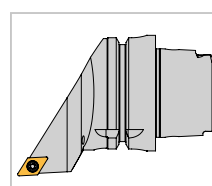
HSK-T63-SDJCL/R 45075-11
