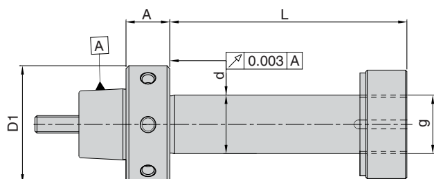
HSK-F40, Ød=20mm
