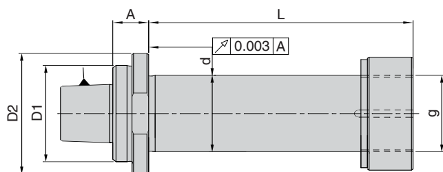
HSK-F40, Ød=31.75mm
