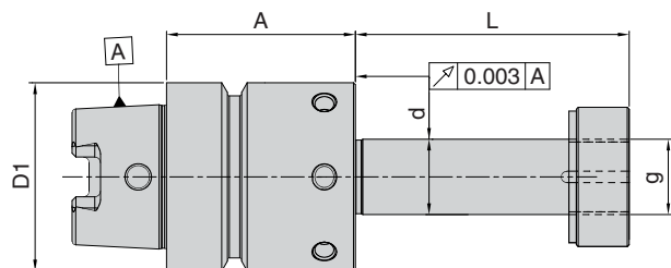
HSK-50, Ød=20mm
