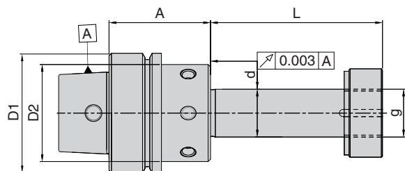
HSK-F50, Ød=20mm
