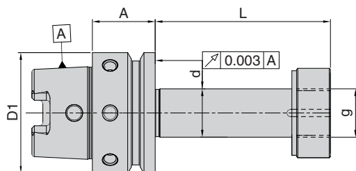
HSK-50 (HSK-C+E50), Ød=20mm
