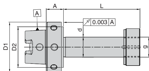
HSK-F40, Ød=20mm
